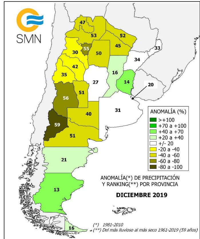
Anomalía (%) y ranking de la precipitación mensual a nivel país y provincial – Diciembre 2019. El sombreado indica la tipificación por rango de anomalía. El número indica la posición en el ranking.
