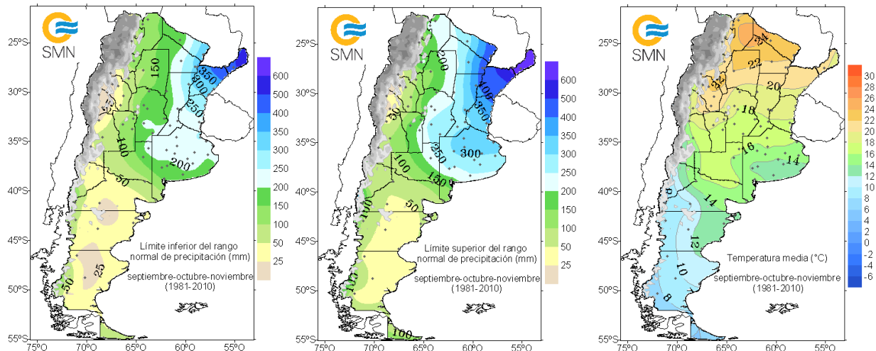
FIG. 9 – Límite inferior del rango normal (mm) (izquierda), límite superior del rango normal (mm) (centro) y temperatura media normal ( ^{\circ}\text{C} ) (derecha) para el trimestre septiembre-octubre-noviembre. Periodo de referencia 1981-2010.
