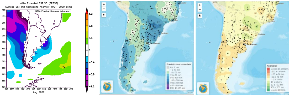
FIG. 8 – Anomalías de la temperatura superficial del mar del agosto de 2022. Período de referencia 1991-2020. Fuente: NOAA. Precipitación acumulada (centro) y anomalía (derecha) (mm) – agosto 2022– Fuente: CRC-SAS
