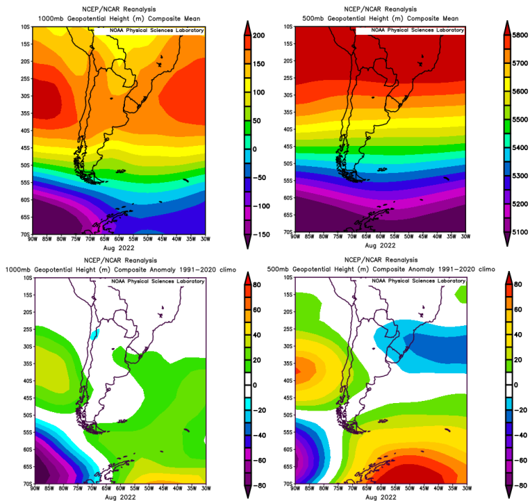
FIG.7– Campo medio de altura geopotencial de la superficie isobárica de 1000 y 500 hPa (arriba) (mgp) y anomalía (abajo) agosto de 2022
