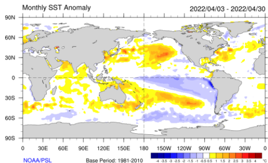
Figura 1 - Anomalías de la temperatura superficial del mar de abril de 2022. Período de referencia 1981-2010. Fuente: NOAA-CIRES/CDC
