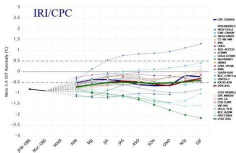
Figura 2 – Pronóstico de anomalías de TSM en la región Niño 3.4. Fuente: IRI.
