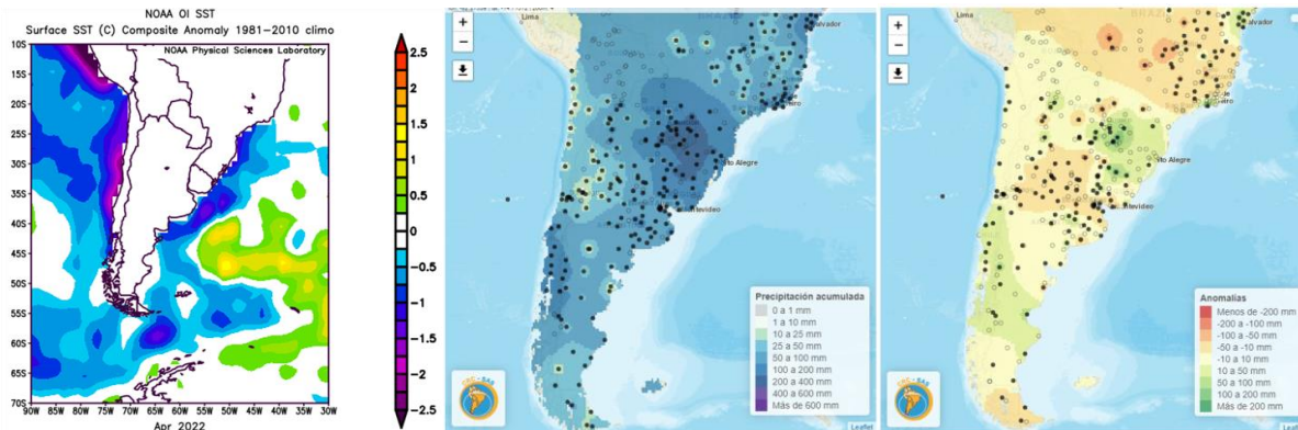
FIG. 8 –Anomalías de la temperatura superficial del mar de abril de 2022. Período de referencia 1981-2010. Fuente: NOAA. Precipitación acumulada (centro) y anomalía (derecha) (mm) – abril 2022– Fuente: CRC-SAS
