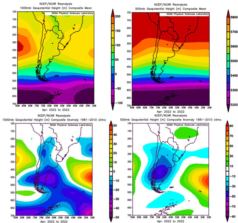
FIG.7- Campo medio de altura geopotencial de la superficie isobárica de 1000 y 500 hPa (arriba) (mgp) y anomalía (abajo) abril de 2022
