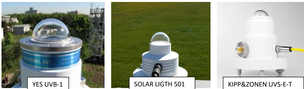
Figura 3. Radiómetros utilizados para medir radiación solar UV en las estaciones del SMN.
