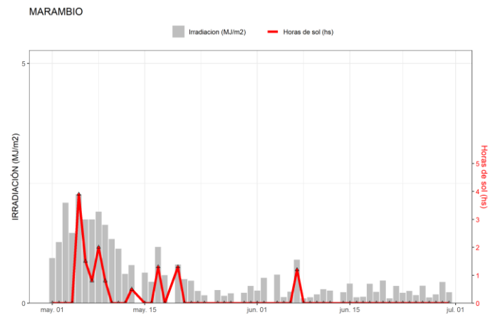
Figura 23. Irradiación solar global diaria y horas de sol obtenidas en Marambio.
