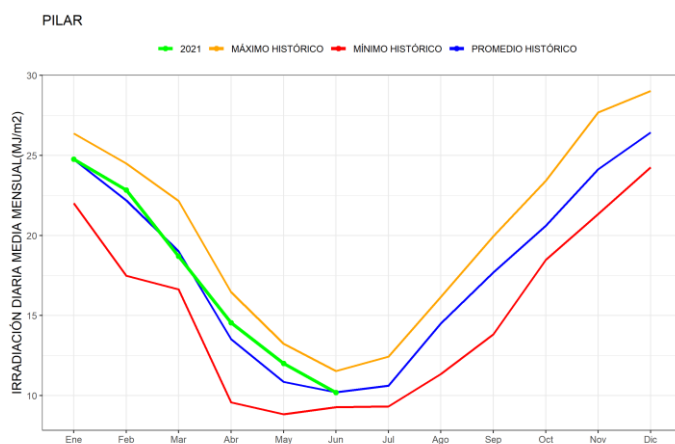
Figura 16. Promedios mensuales de irradiación solar global diaria junto con los valores históricos disponibles de Pilar
