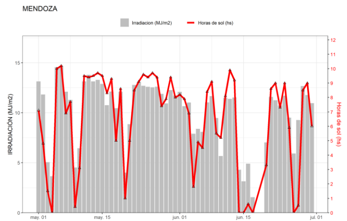
Figura 25. Irradiación solar global diaria y horas de sol obtenidas en Mendoza.
