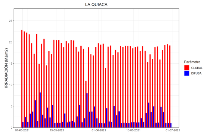
Figura 5. Irradiación solar global y difusa diaria disponibles para La Quiaca durante el bimestre considerado
