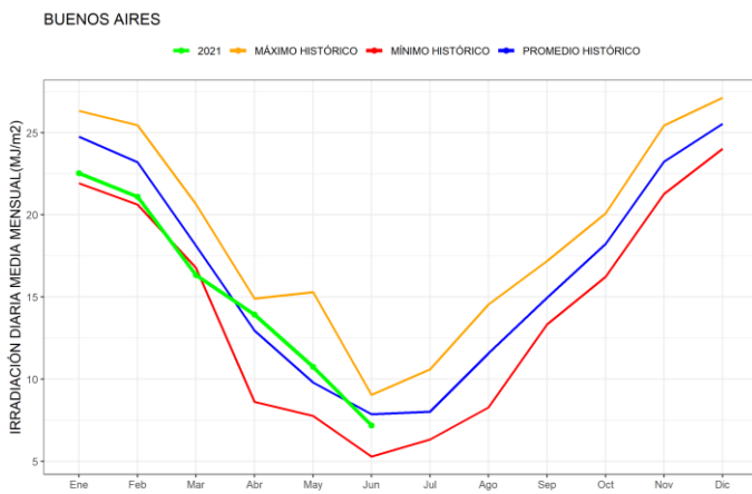
Figura 14. Promedios mensuales de irradiación solar global diaria junto con los valores históricos disponibles de Buenos Aires
