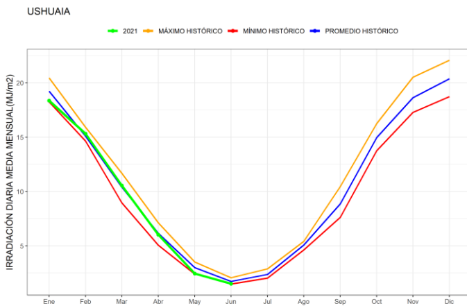
Figura 18. Promedios mensuales de irradiación solar global diaria junto con los valores históricos disponibles de Ushuaia
