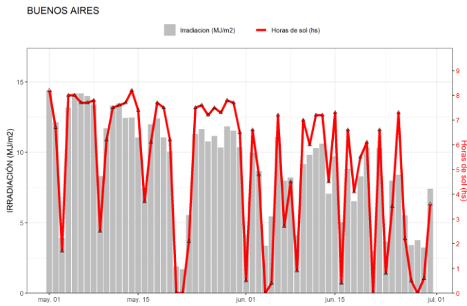
Figura 20. Irradiación solar global diaria y horas de sol obtenidas en Buenos Aires.
