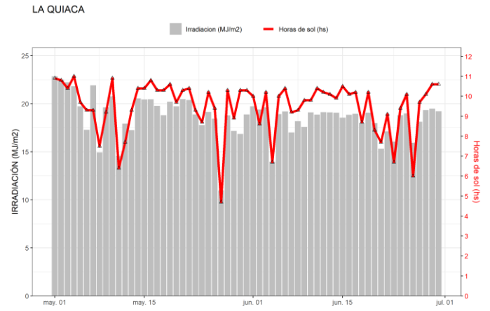
Figura 21. Irradiación solar global diaria y horas de sol obtenidas en La Quiaca.
