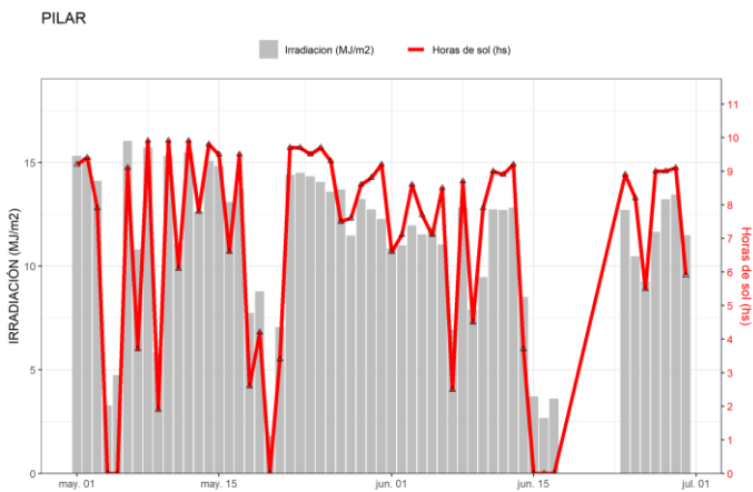
Figura 22. Irradiación solar global diaria y horas de sol obtenidas en Pilar.
