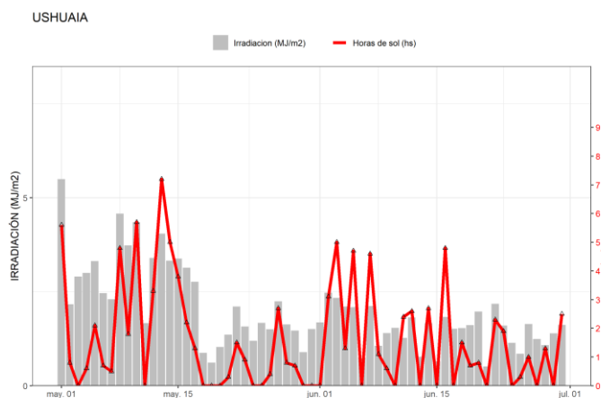
Figura 24. Irradiación solar global diaria y horas de sol obtenidas en Ushuaia.
