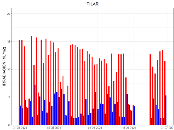
Figura 4. Irradiación solar global y difusa diaria disponibles para Pilar durante el bimestre considerado
