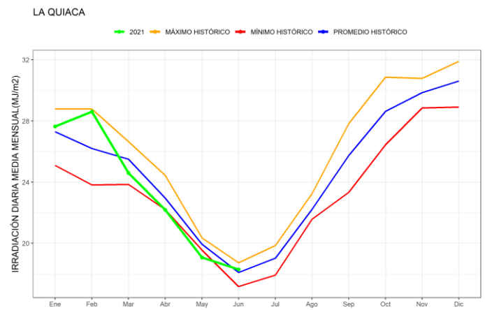
Figura 15. Promedios mensuales de irradiación solar global diaria junto con los valores históricos disponibles de La Quiaca
