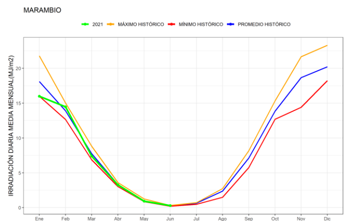
Figura 17. Promedios mensuales de irradiación solar global diaria junto con los valores históricos disponibles de Marambio
