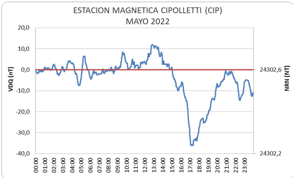
Figura 8: Variación Diaria Perturbada del mes de mayo
