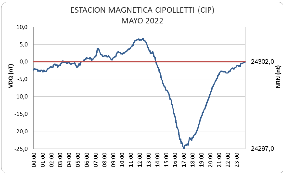
Figura 7: Variación Diaria Calma del mes de mayo
