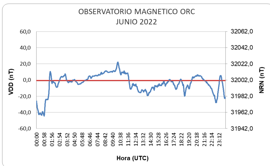
Figura 9: Variación Diaria Perturbada del mes de junio
