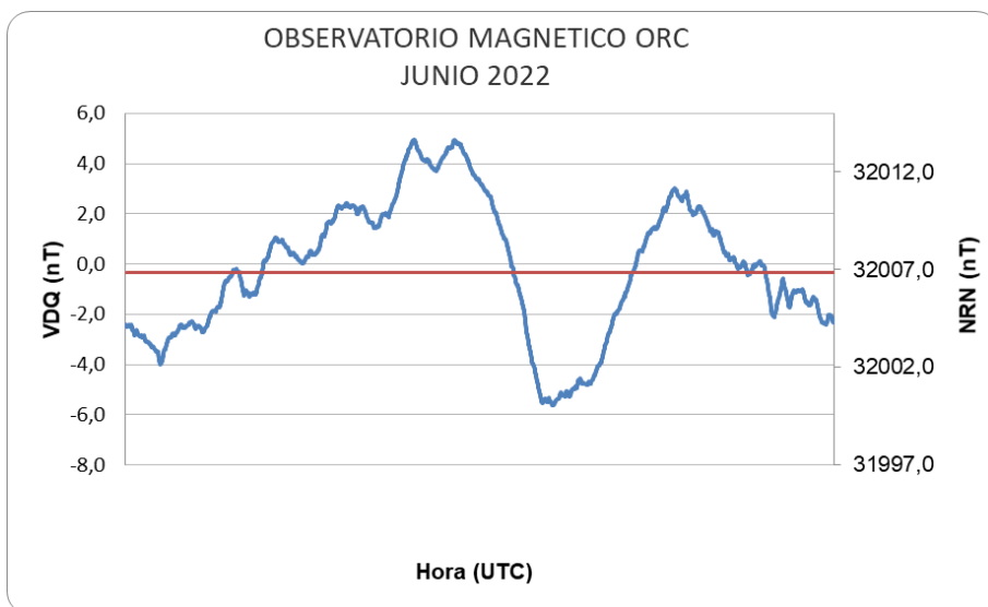
Figura 8: Variación Diaria Calma del mes de junio
