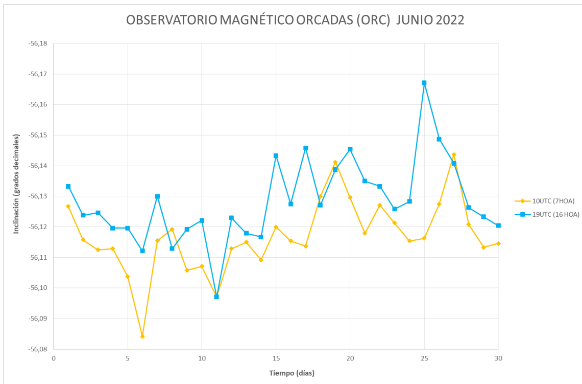
Figura 6: Inclínación magnética en función del tiempo
