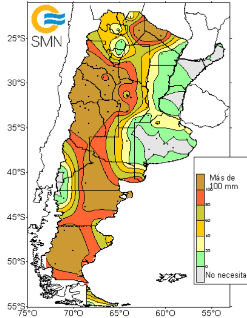
Agua necesaria para no estar en Comienzo de Sequia en los próximos 10 días a partir del 31 de mayo de 2022
