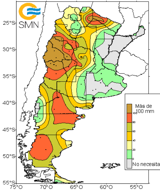
Agua necesaria para no estar en Sequia en los próximos 10 días a partir del 31 de mayo de 2022
