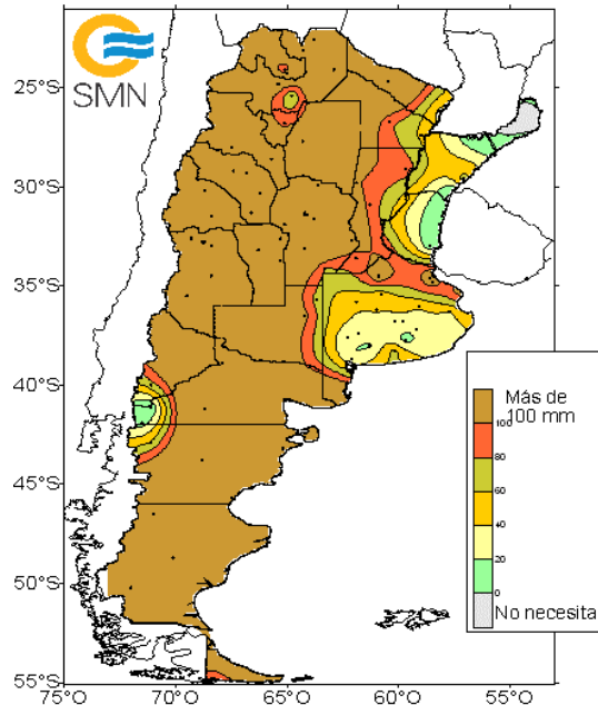
Agua necesaria para comenzar a tener Excesos en los próximos 10 días a partir del 31 de mayo de 2022
