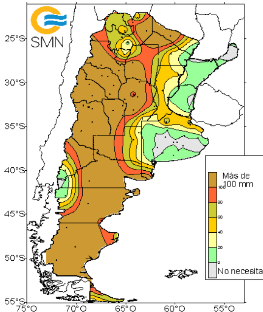
Agua necesaria para tener Buenas Condiciones en los próximos 10 días a partir del 31 de mayo de 2022
