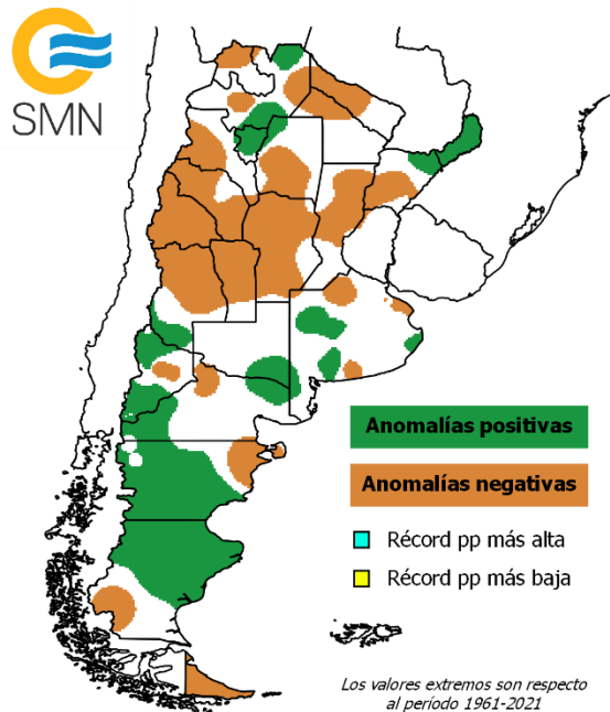
Precipitación - abril 2022
