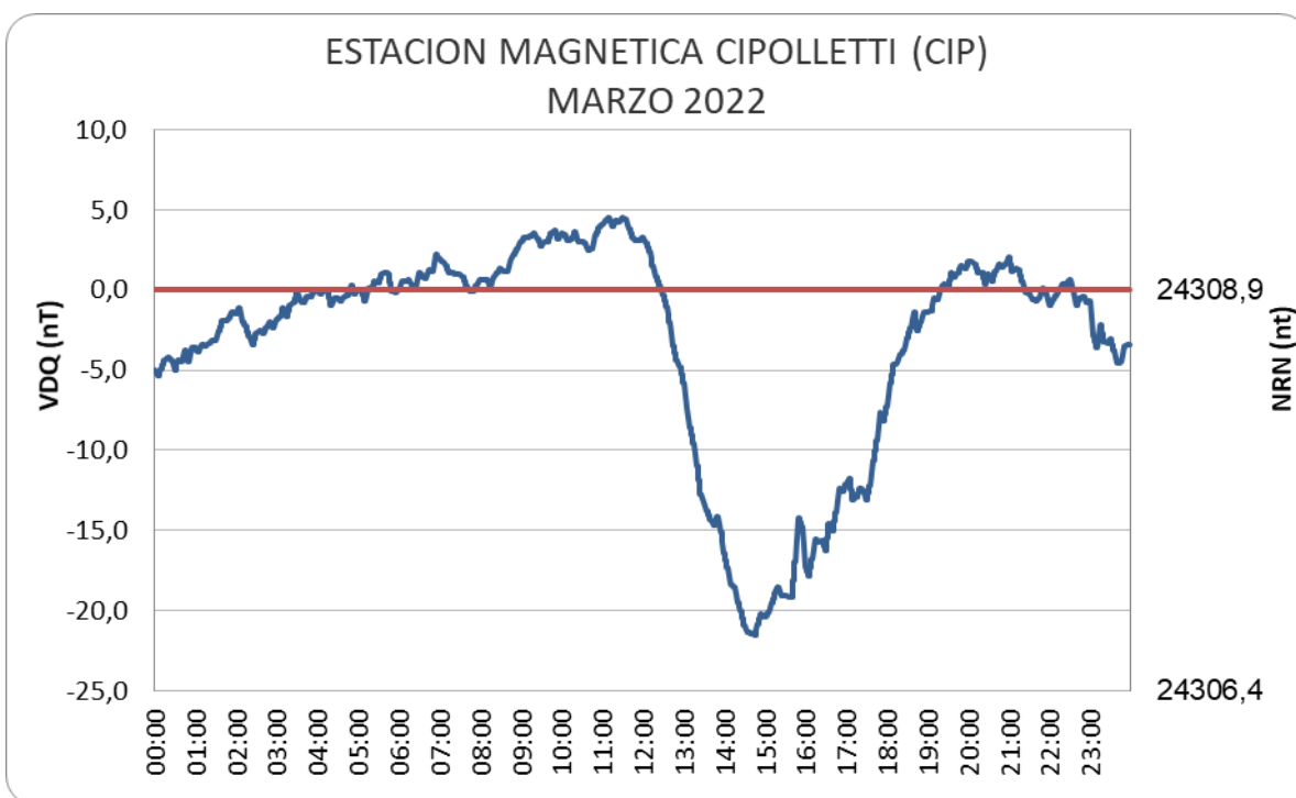
Figura 7: Variación Diaria Calma del mes de marzo
