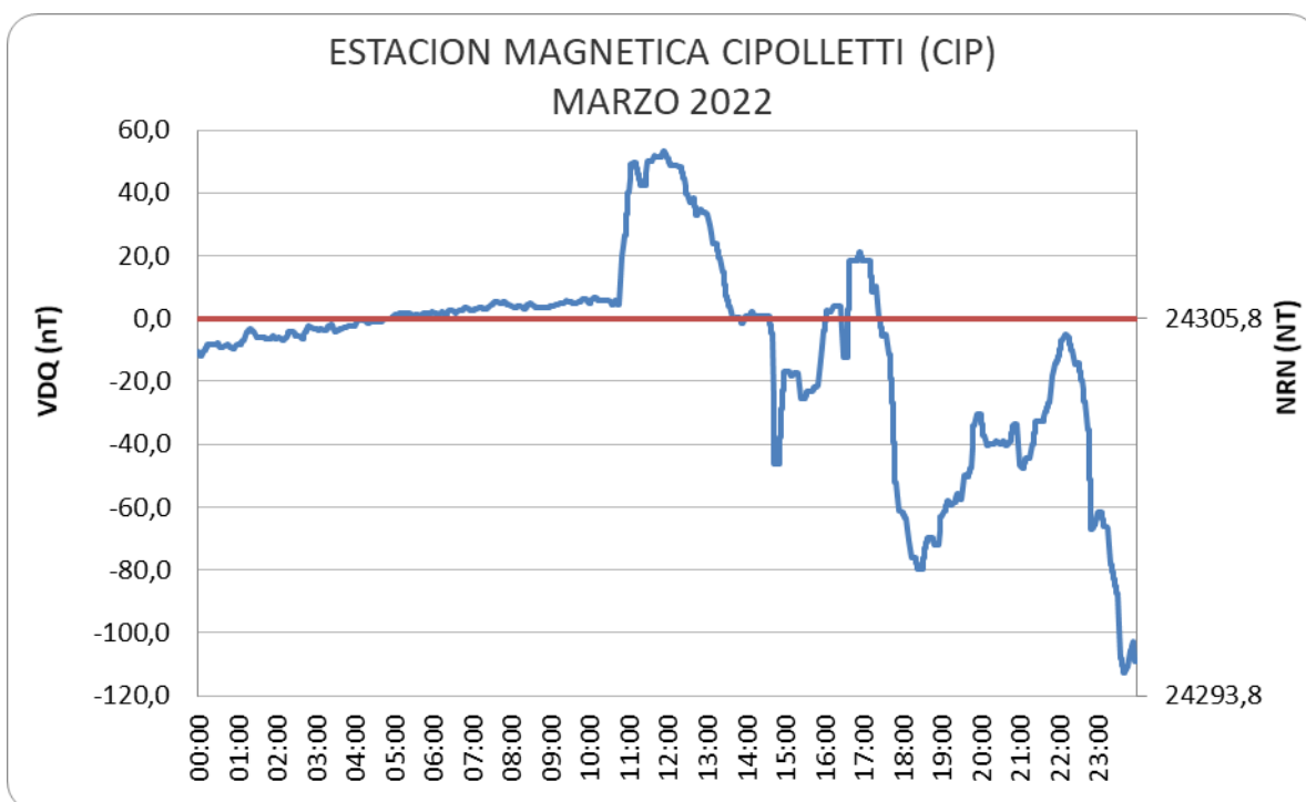
Figura 8: Variación Diaria Perturbada del mes de marzo
