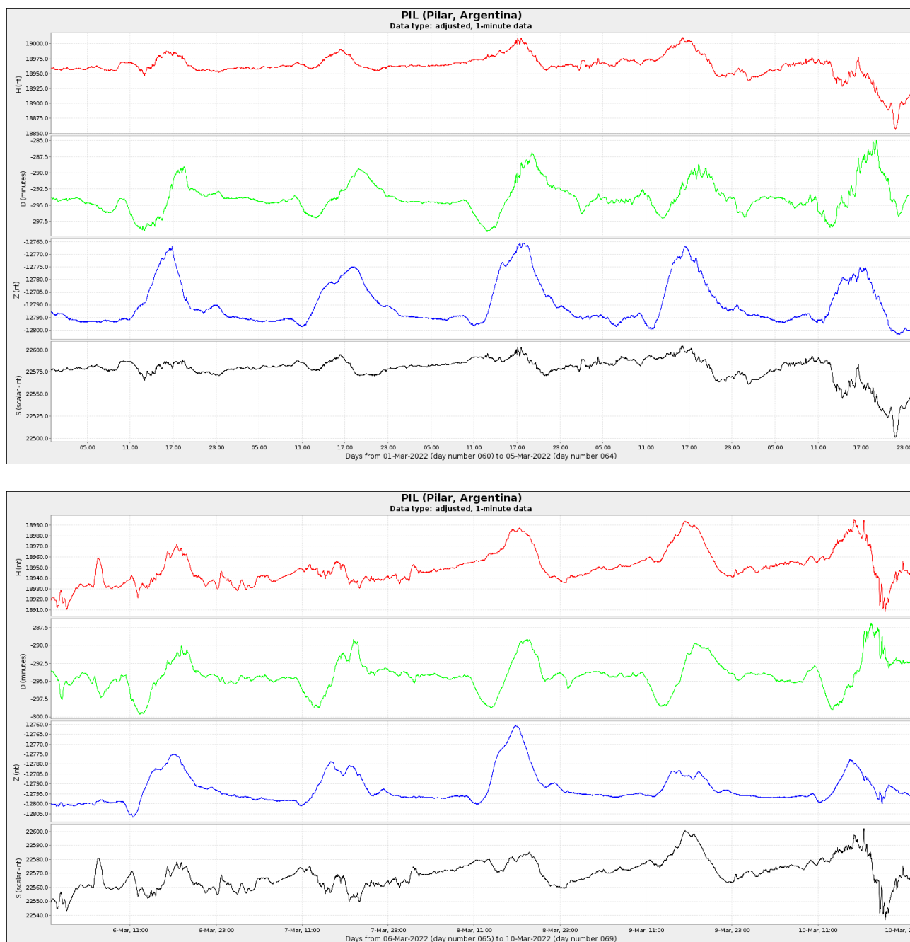
Figura 4a: Componentes del campo magnético del día 1 al 10 de marzo. En rojo se ve la componente horizontal (H) y en azul la vertical (Z), ambas en nT. En verde se presenta la declinación del campo magnético (D) en minutos y en negro la intensidad del campo magnético en nT
