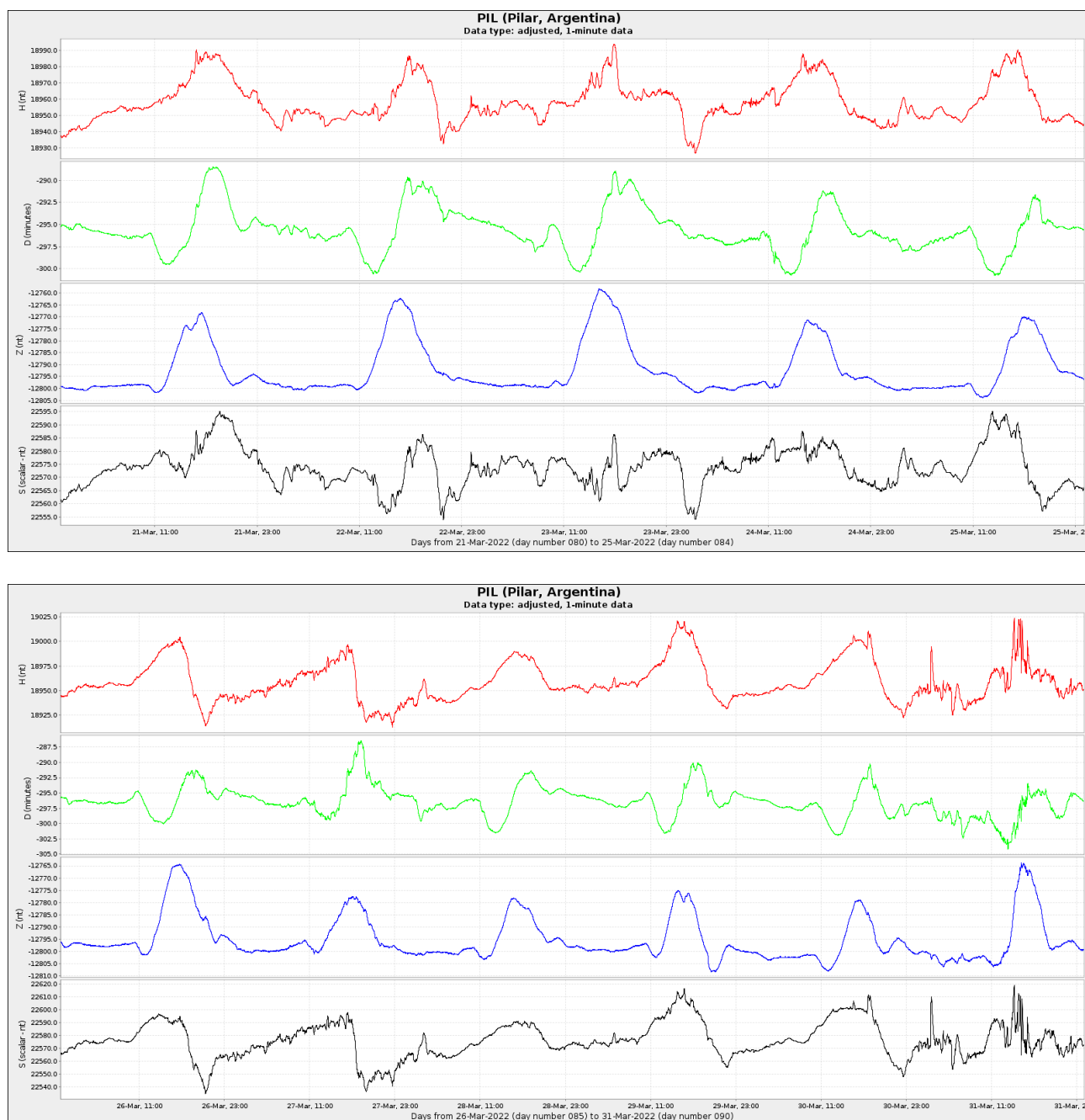
Figura 4c: Componentes del campo magnético del 21 al 31 de marzo. En rojo se ve la componente horizontal (H) y en azul la vertical (Z), ambas en nT. En verde se presenta la declinación del campo magnético (D) en minutos y en negro la intensidad del campo magnético en nT.
