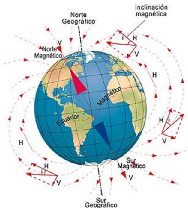
Figura 2: Representación gráfica del campo magnético terrestre
