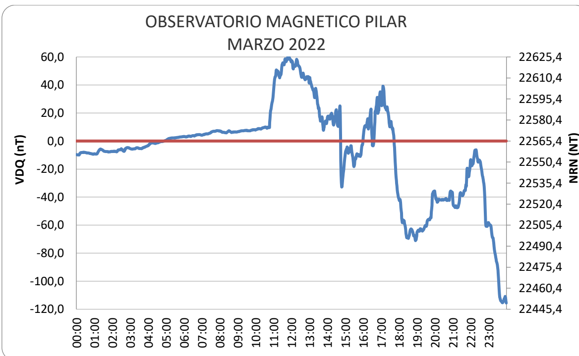
Figura 9: Variación Diaria Perturbada del mes de marzo
