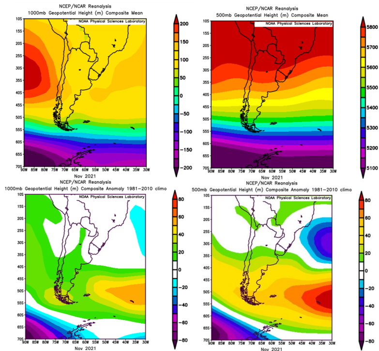
FIG.7- Campo medio de altura geopotencial de la superficie isobárica de 1000 y 500 hPa (arriba) (mgp) y anomalía (abajo) noviembre 2021
