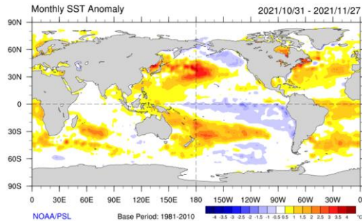
Figura 1 - Anomalías de la temperatura superficial del mar de noviembre de 2021. Período de referencia 1981-2010. Fuente: NOAA-CIRES/CDC
