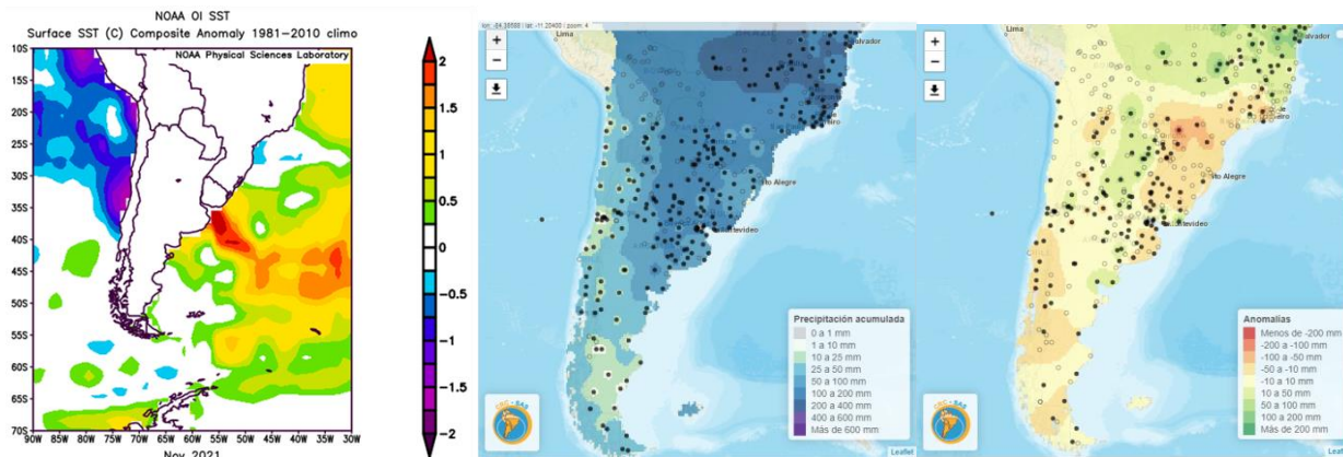
FIG. 8—Anomalías de la temperatura superficial del mar noviembre 2021. Período de referencia 1981–2010. Fuente: NOAA. Precipitación acumulada (centro) y anomalía (derecha) (mm) – noviembre 2021—Fuente: CRC-SAS
