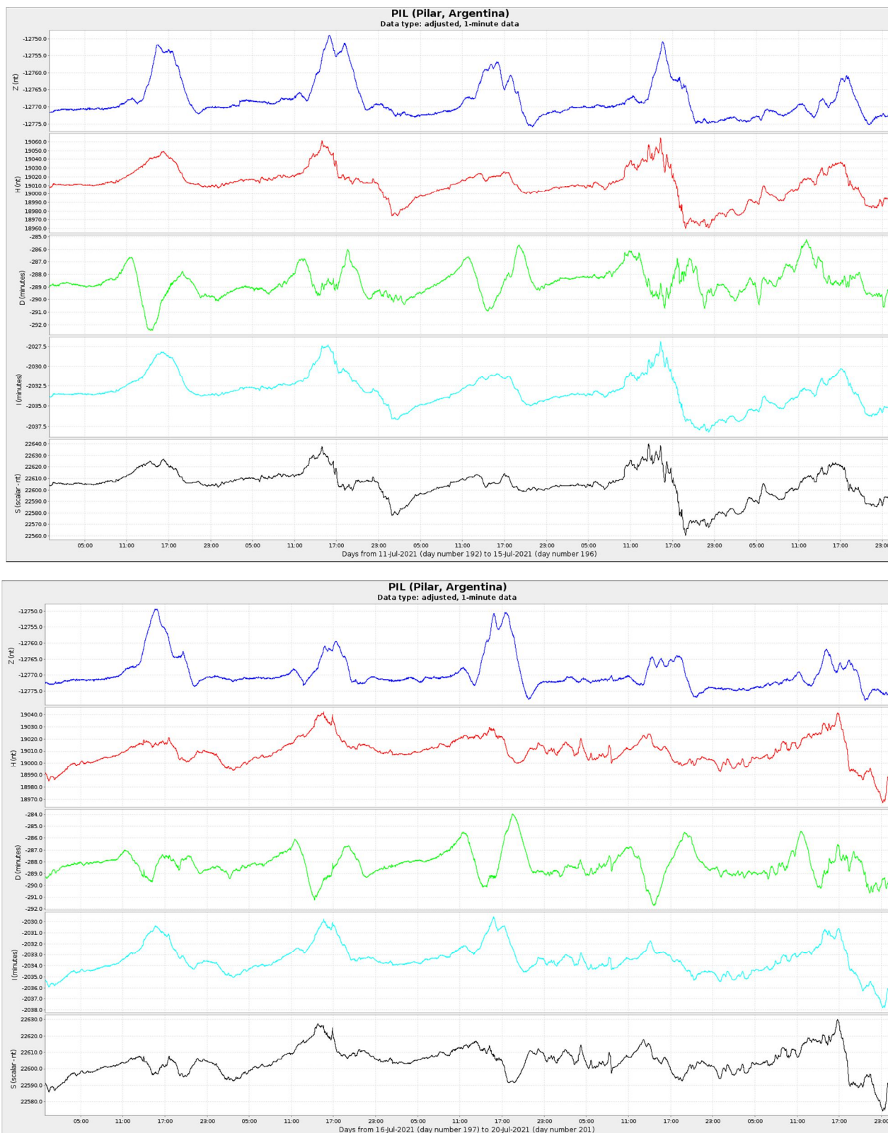
Figura 4b: Componentes del campo magnético del 11 al 20 de julio. En rojo se ve la componente horizontal (H) y en azul la vertical (Z), ambas en nT. En verde se presenta la declinación del campo magnético (D) en minutos y en negro la intensidad del campo magnético en nT.
