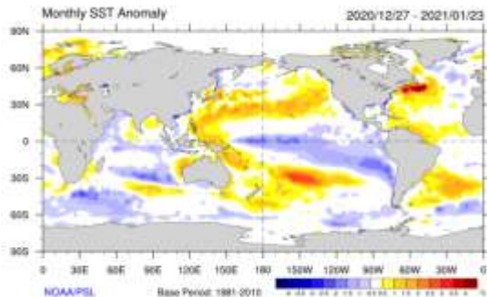
Figura 1 - Anomalías de la temperatura superficial del mar de enero de 2021. Período de referencia 1981-2010. Fuente: NOAA-CIRES/CDC
