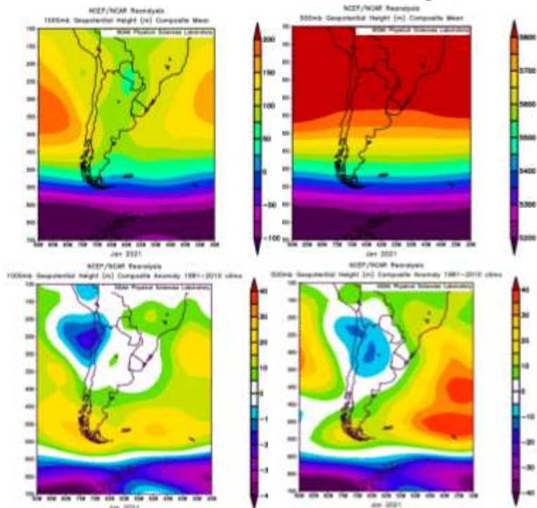
FIG.7– Campo medio de altura geopotencial de la superficie isobárica de 1000 y 500 hPa (arriba) (m) y anomalía (abajo) enero de 2021
