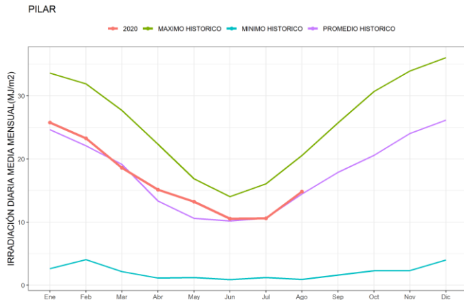
Figura 26. Promedios mensuales de irradiación solar global diaria junto con los valores históricos disponibles de Pilar
