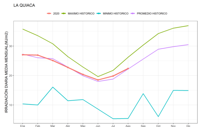
Figura 25. Promedios mensuales de irradiación solar global diaria junto con los valores históricos disponibles de La Quiaca
