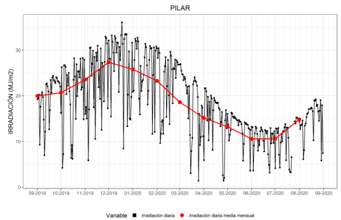
Figura 16. Irradiación solar global diaria y promedios mensuales de los últimos 12 meses en Pilar.
