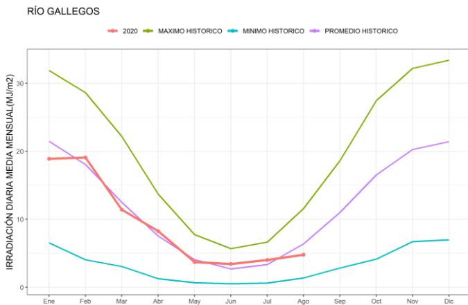
Figura 22. Promedios mensuales de irradiación solar global diaria junto con los valores históricos disponibles de Río Gallegos
