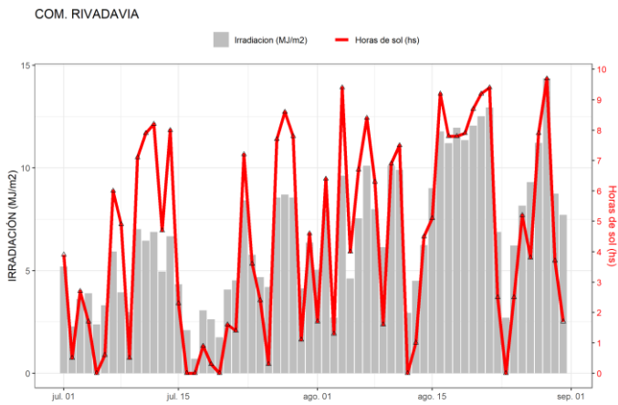
Figura 35. Irradiación solar global diaria y horas de sol obtenidas en Com. Rivadavia.
