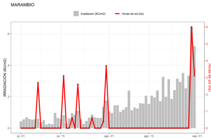
Figura 33. Irradiación solar global diaria y horas de sol obtenidas en Marambio.
