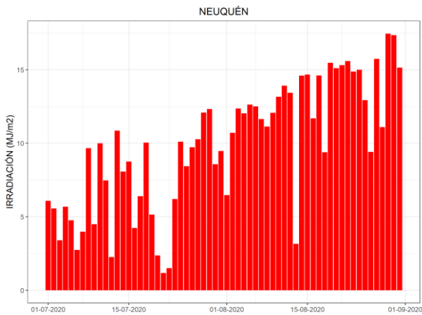
Figura 9. Irradiación solar global diaria disponible para Neuquén durante el bimestre considerado
