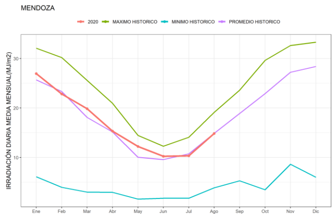
Figura 23. Promedios mensuales de irradiación solar global diaria junto con los valores históricos disponibles de Mendoza
