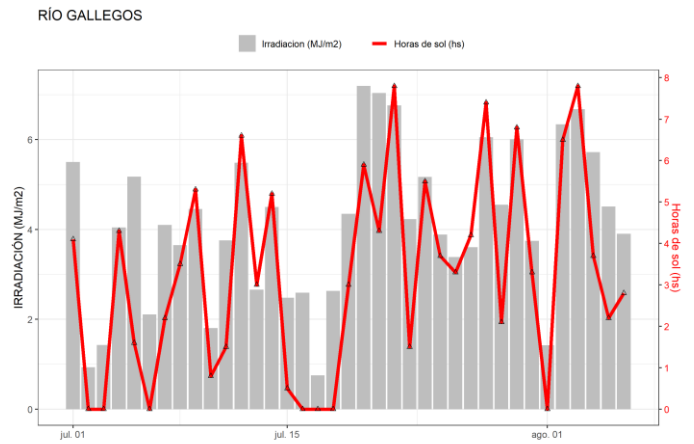
Figura 36. Irradiación solar global diaria y horas de sol obtenidas en Río Gallegos.
