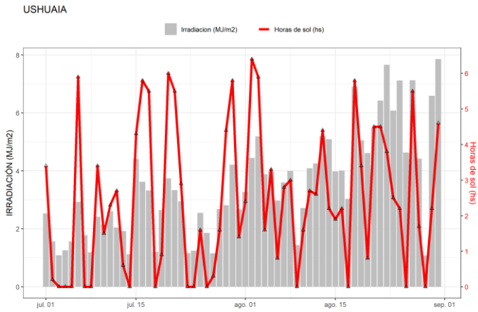
Figura 29. Irradiación solar global diaria y horas de sol obtenidas en Ushuaia.
