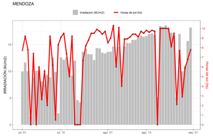
Figura 30. Irradiación solar global diaria y horas de sol obtenidas en Mendoza.
