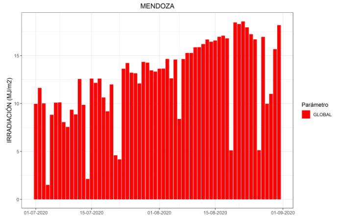
Figura 4. Irradiación solar global diaria disponible para Mendoza durante el bimestre considerado
