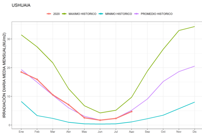
Figura 28. Promedios mensuales de irradiación solar global diaria junto con los valores históricos disponibles de Ushuaia
