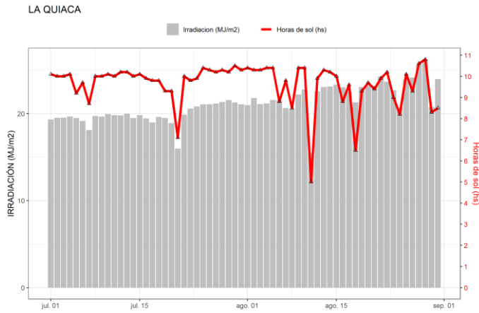
Figura 31. Irradiación solar global diaria y horas de sol obtenidas en La Quiaca.
