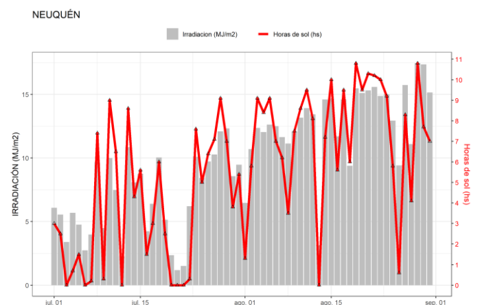
Figura 34. Irradiación solar global diaria y horas de sol obtenidas en Neuquén.
