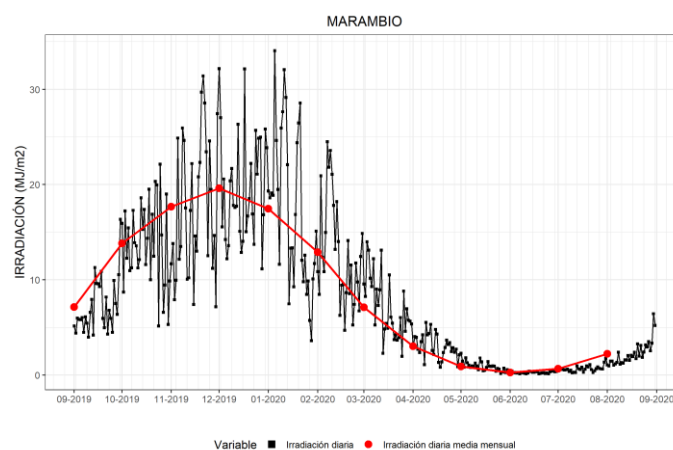
Figura 17. Irradiación solar global diaria y promedios mensuales de los últimos 12 meses en Marambio.
