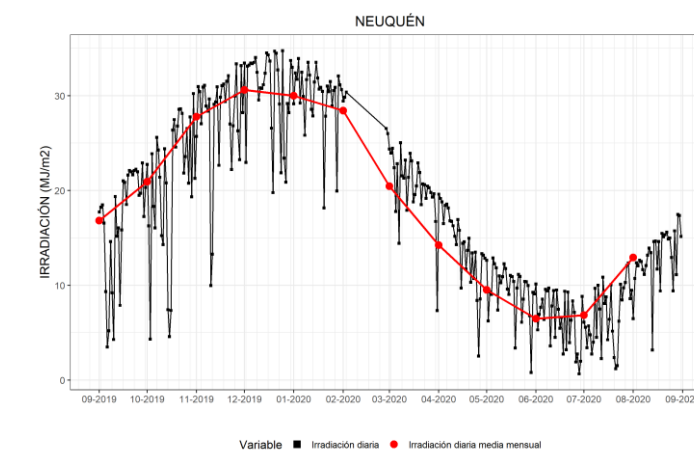
Figura 18. Irradiación solar global diaria y promedios mensuales de los últimos 12 meses en Neuquén.
