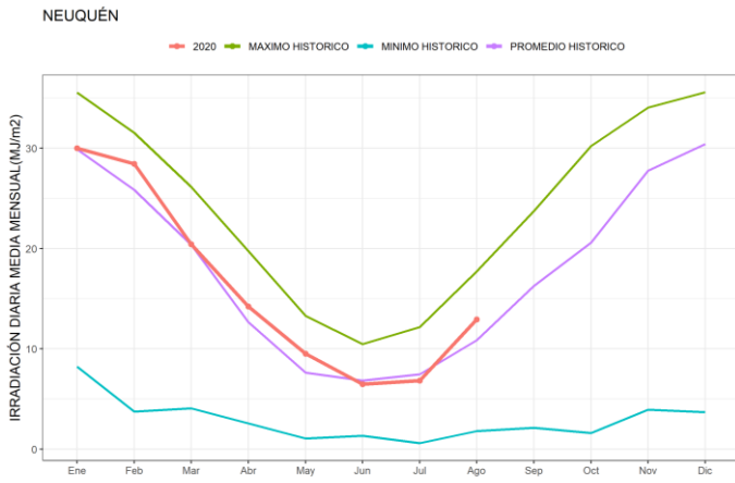
Figura 20. Promedios mensuales de irradiación solar global diaria junto con los valores históricos disponibles de Neuquén
