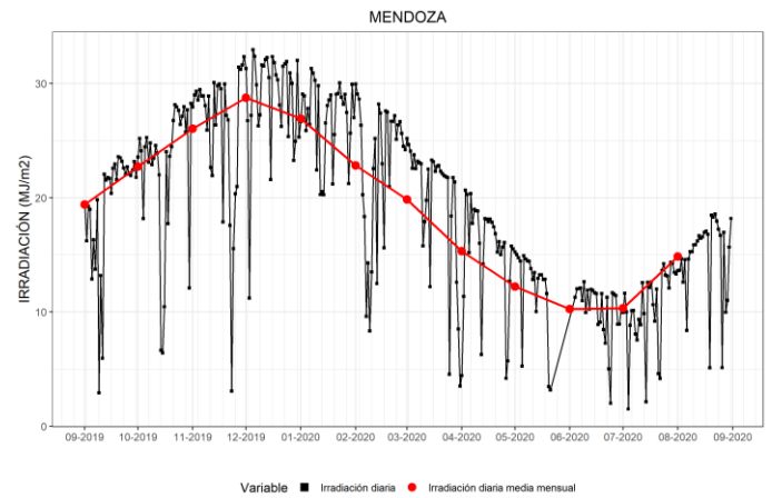
Figura 14. Irradiación solar global diaria y promedios mensuales de los últimos 12 meses en Mendoza.
