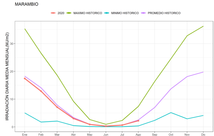
Figura 27. Promedios mensuales de irradiación solar global diaria junto con los valores históricos disponibles de Marambio
