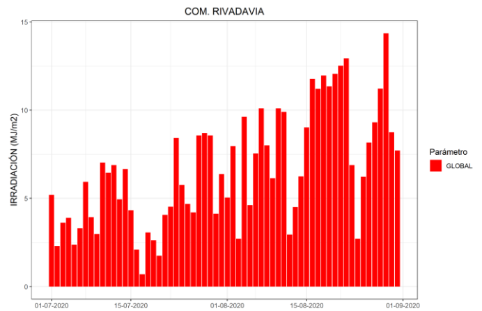
Figura 10. Irradiación solar global diaria disponible para Com. Rivadavia durante el bimestre considerado
