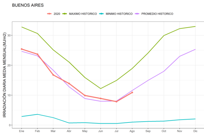
Figura 24. Promedios mensuales de irradiación solar global diaria junto con los valores históricos disponibles de Buenos Aires
