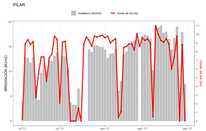
Figura 32. Irradiación solar global diaria y horas de sol obtenidas en Pilar.
