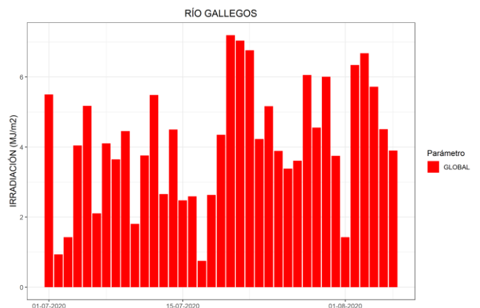
Figura 8. Irradiación solar global diaria disponible para Río Gallegos durante el bimestre considerado
