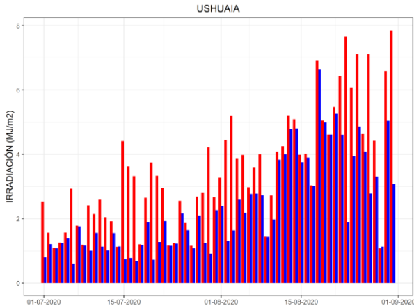
Figura 3. Irradiación solar global y difusa diaria disponible para Ushuaia durante el bimestre considerado
