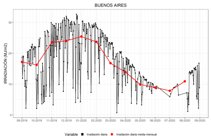
Figura 12. Irradiación solar global diaria y promedios mensuales de los últimos 12 meses en Buenos Aires.
