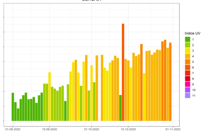
Figura 11. Índice UV máximo diario medido en Ushuaia
