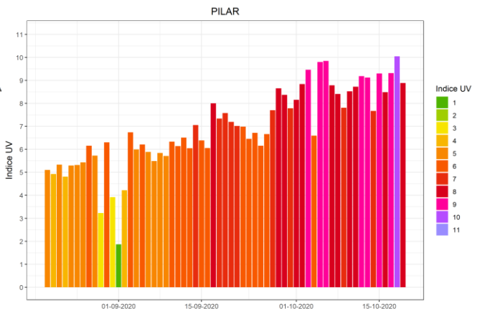
Figura 5. Índice UV máximo diario medido en Pilar
