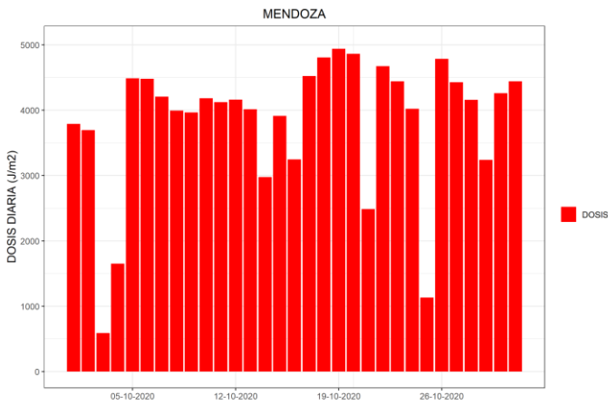
Figura 14. Índice UV máximo diario medido en Mendoza
