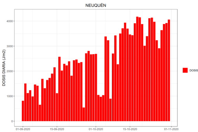
Figura 16. Índice UV máximo diario medido en Neuquén
