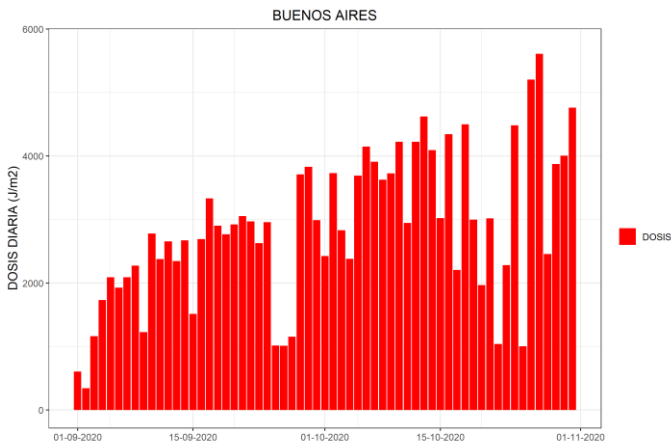
Figura 12. Índice UV máximo diario medido en Buenos Aires
