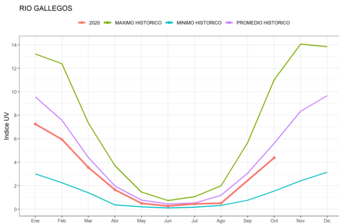
Figura 34. Promedios mensuales de índice UV máximo diario junto con los valores históricos disponibles de Rio Gallegos
