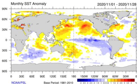
Figura 1 - Anomalías de la temperatura superficial del mar de noviembre de 2020. Período de referencia 1981-2010. Fuente: NOAA-CIRES/CDC
