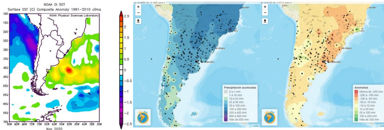
FIG. 8 –Anomalías de la temperatura superficial del mar noviembre de 2020. Período de referencia 1981-2010. Fuente: NOAA. Precipitación acumulada (centro) y anomalía (derecha) (mm) – noviembre 2020 – Fuente: CRC-SAS
