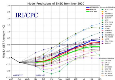
Figura 2 – Pronóstico de anomalías de TSM en la región Niña
