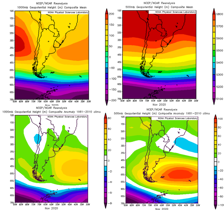
FIG.7- Campo medio de altura geopotencial de la superficie isobárica de 1000 y 500 hPa (arriba) (m) y anomalía (abajo) noviembre de 2020
