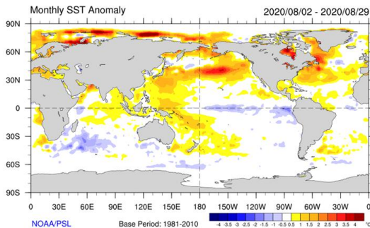
Figura 1 - Anomalías de la temperatura superficial del mar de agosto de 2020. Período de referencia 1981-2010. Fuente: NOAA-CIRES/CDC
