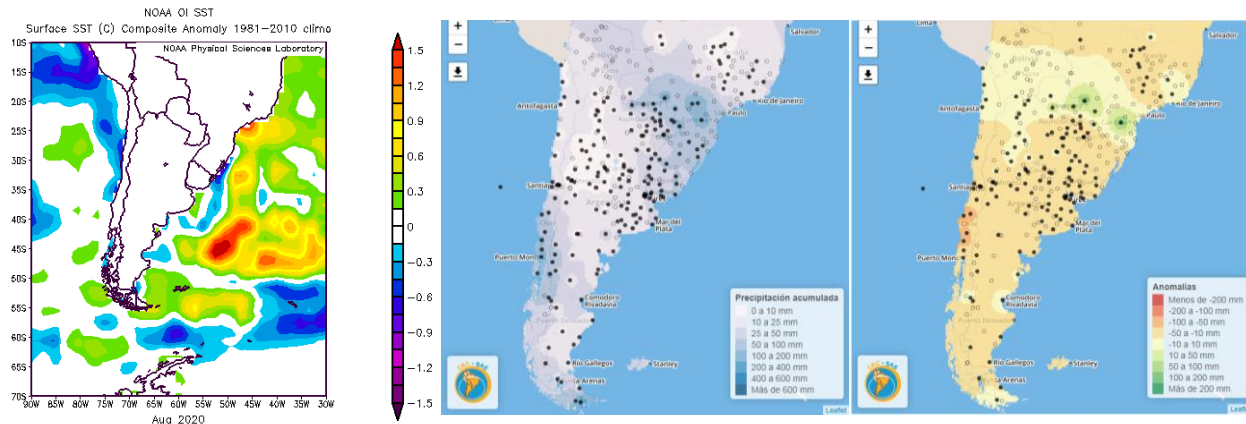
FIG. 8 –Anomalías de la temperatura superficial del mar de agosto de 2020. Período de referencia 1981–2010. Fuente: NOAA. Precipitación acumulada (centro) y anomalía (derecha) (mm) – agosto 2020 – Fuente: CRC-SAS
