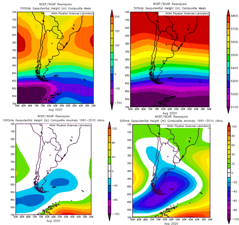
FIG.7– Campo medio de altura geopotencial de la superficie isobárica de 1000 y 500 hPa (arriba) (mgp) y anomalía (abajo) agosto de 2020
