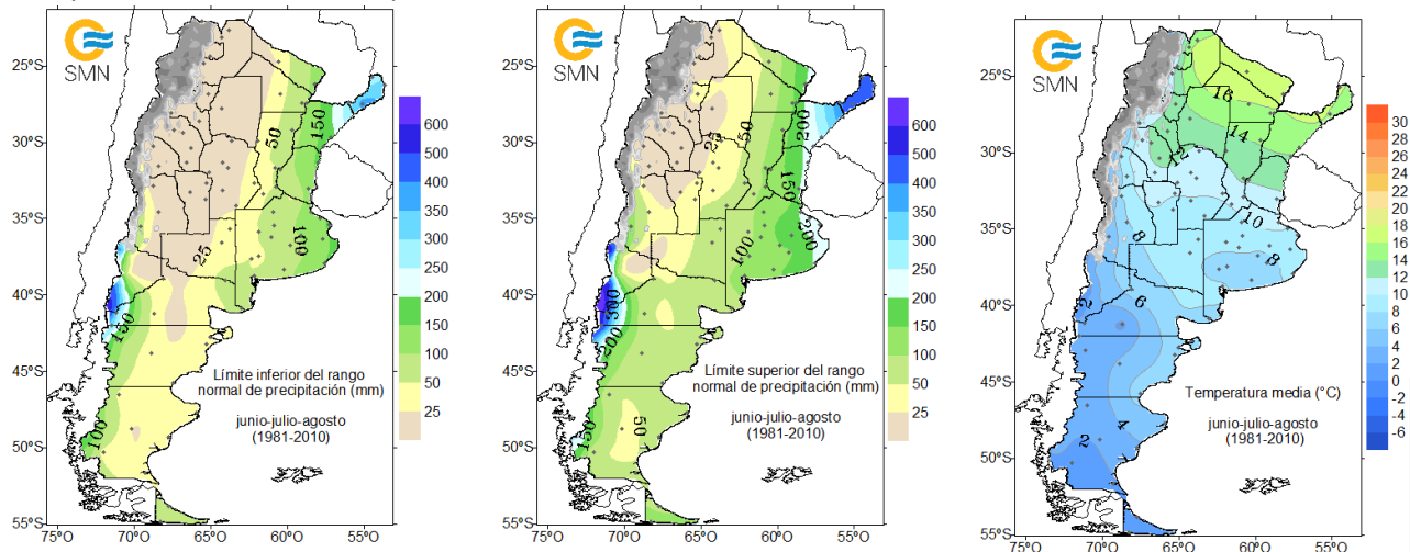
FIG. 9 – Límite inferior del rango normal (mm) (izquierda), límite superior del rango normal (mm) (centro) y temperatura media normal (°C) (derecha) para el trimestre junio-julio-agosto. Período de referencia 1981-2010.
