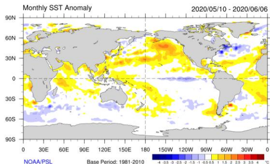
Figura 1 - Anomalías de la temperatura superficial del mar de mayo de 2020. Período de referencia 1981-2010. Fuente: NOAA-CIRES/CDC
