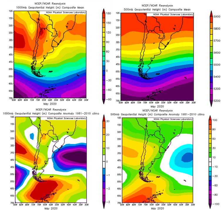
FIG.7– Campo medio de altura geopotencial de la superficie isobárica de 1000 y 500 hPa (arriba) (m) y anomalía (abajo) mayo de 2020
