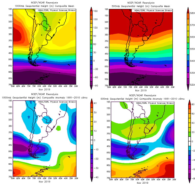
FIG.7– Campo medio de altura geopotencial de la superficie isobárica de 1000 y 500 hPa (arriba) (mgp) y anomalía (abajo) noviembre 2019
