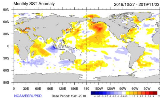
Figura 1 - Anomalías de la temperatura superficial del mar de noviembre de 2019. Período de referencia 1981-2010. Fuente: NOAA-CIRES/CDC
