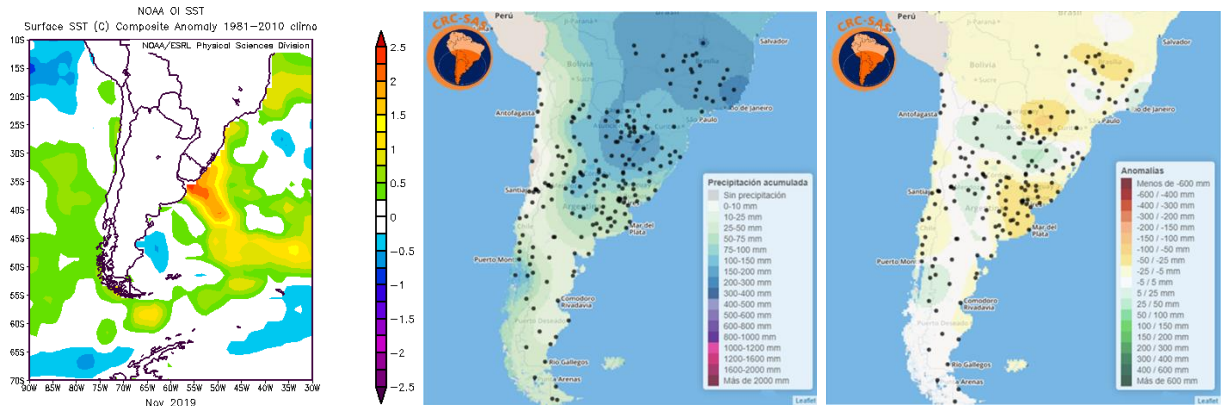
FIG. 8 –Anomalías de la temperatura superficial del mar de noviembre de 2019. Período de referencia 1981-2010. Fuente: NOAA. Precipitación acumulada (centro) y anomalía (derecha) (mm) –noviembre 2019 – Fuente: CRC-SAS
