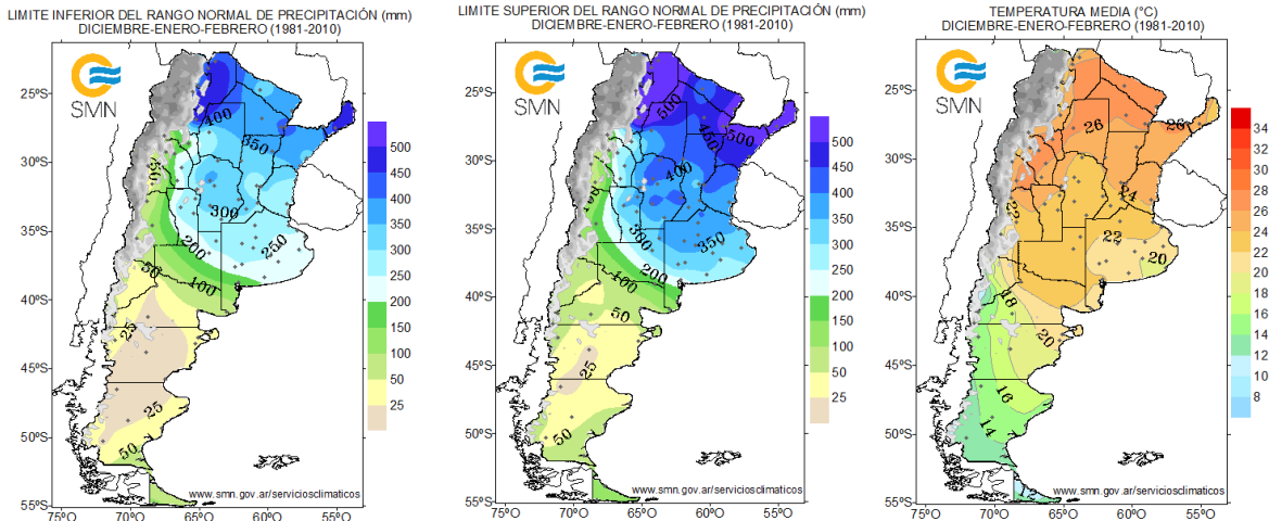
FIG. 9 – Límite inferior del rango normal (mm) (izquierda), límite superior del rango normal (mm) (centro) y temperatura media normal ( ^{\circ}\text{C} ) (derecha) para el trimestre diciembre-enero-febrero. Período de referencia 1981-2010.
