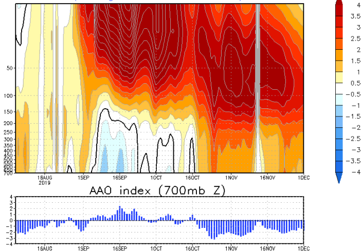
FIG. 3 – Evolución temporal de la anomalía normalizada de geopotencial entre 65°S y 90°S (arriba) y del índice OA (abajo) Fuente: NCEP/NOAA
