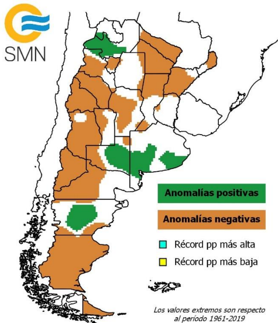
Precipitación - Abril 2020
