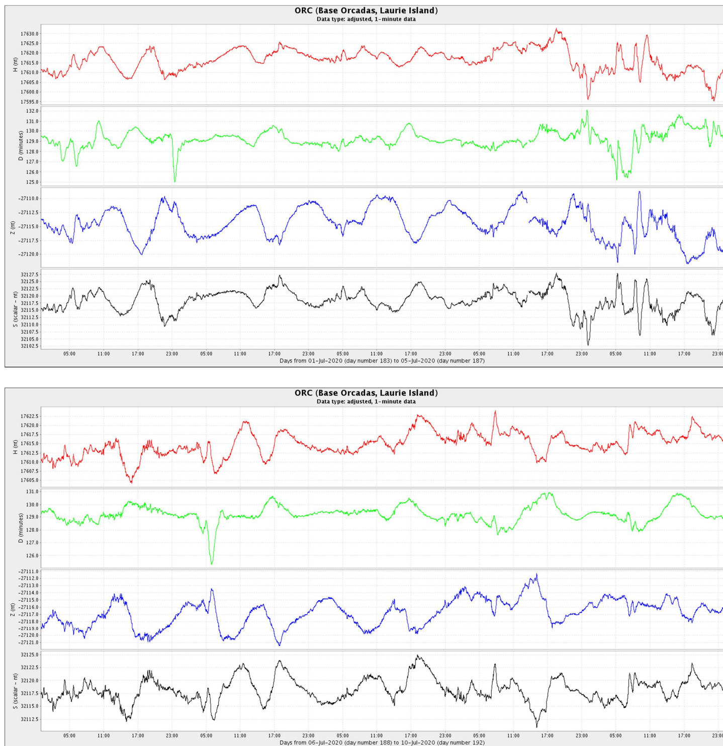
Figura 4a: Componentes del campo magnético del 1 al 10 de julio. En rojo se ve la componente horizontal (H) y en azul la vertical (Z), ambas en nT. En verde se presenta la declinación del campo magnético (D) en minutos y en negro la intensidad del campo magnético en nT
