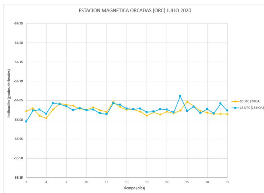
Figura 6: Inclinación magnética en función del tiempo
