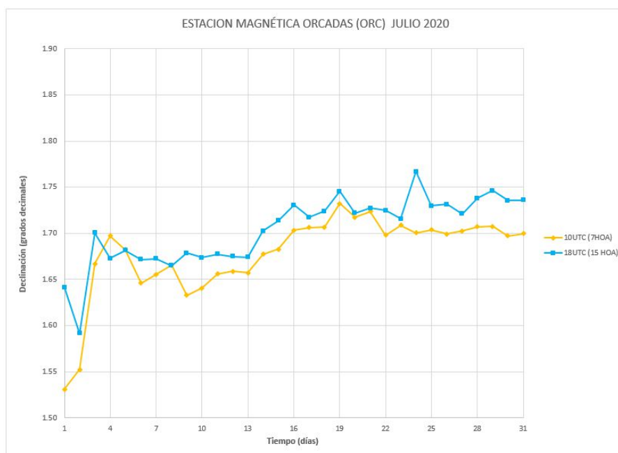
Figura 5: Declinación magnética en función del tiempo
