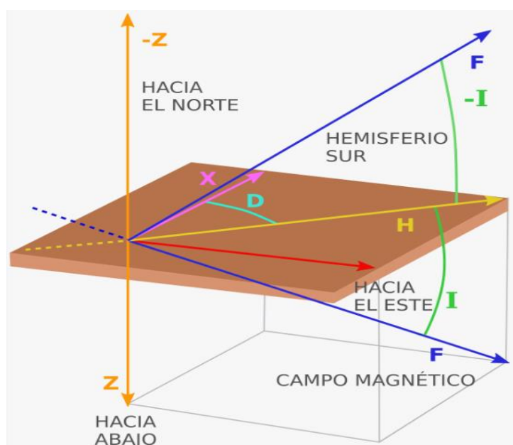
Figura 3: Componentes del campo magnético
