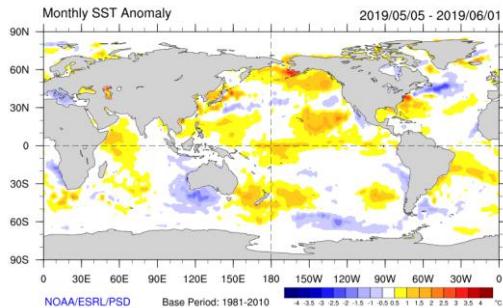
Figura 1 - Anomalías de la temperatura superficial del mar de mayo de 2019. Período de referencia 1981-2010. Fuente: NOAA-CIRES/CDC
