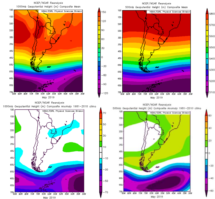
FIG.7– Campo medio de altura geopotencial de la superficie isobárica de 1000 y 500 hPa (arriba) (m) y anomalía (abajo) mayo 2019
