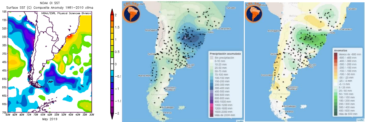
FIG. 8 – Anomalías de la temperatura superficial del mar de mayo de 2019. Período de referencia 1981-2010. Fuente: NOAA. Precipitación acumulada (centro) y anomalía (derecha) (mm) – mayo 2019 – Fuente: CRC-SAS
